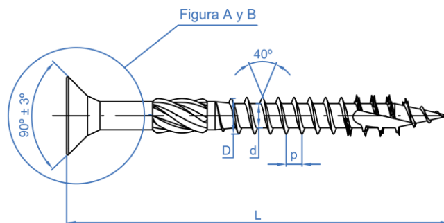
Figura A: avellanado interior 2.5 ÷ 4.5
